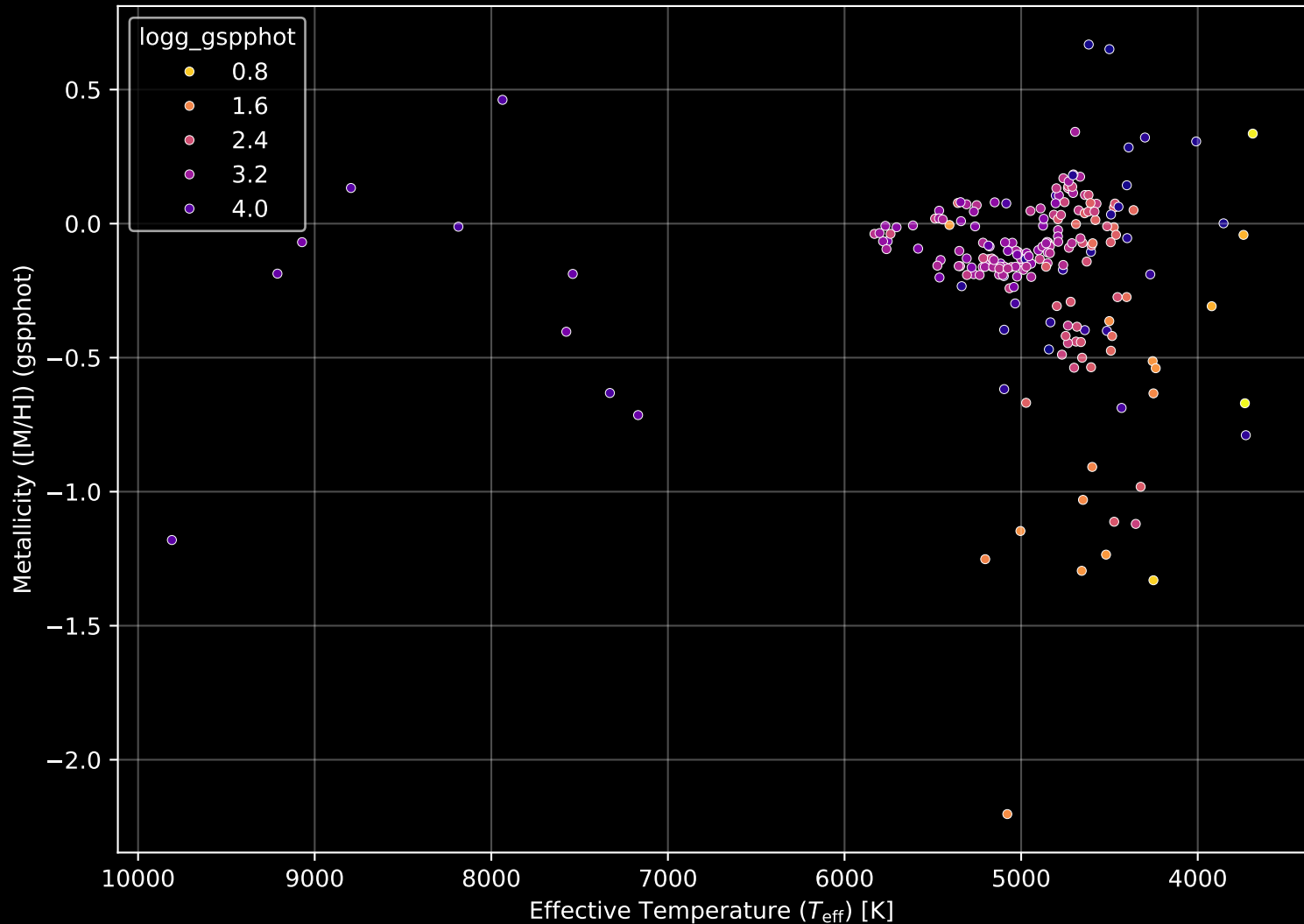
APOGEE DR17 Field: [311-12] Stellar Population Parameters (n= 210)
